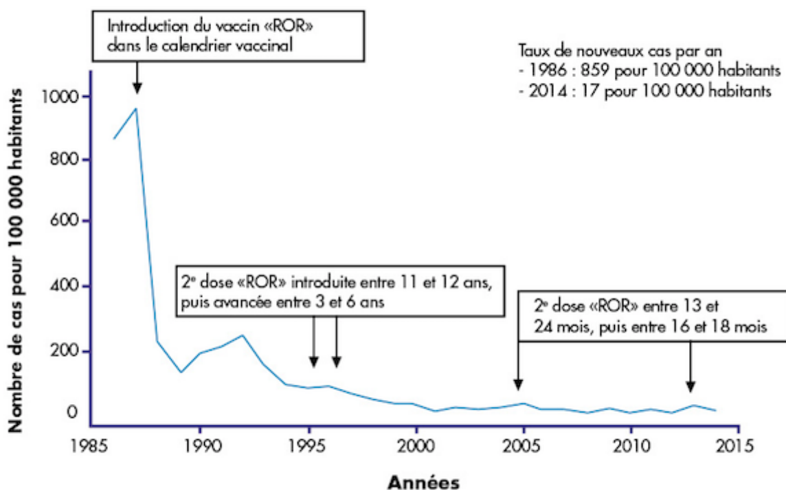
Oreillons : nombre de cas par an, en France, de 1985 à 2015
